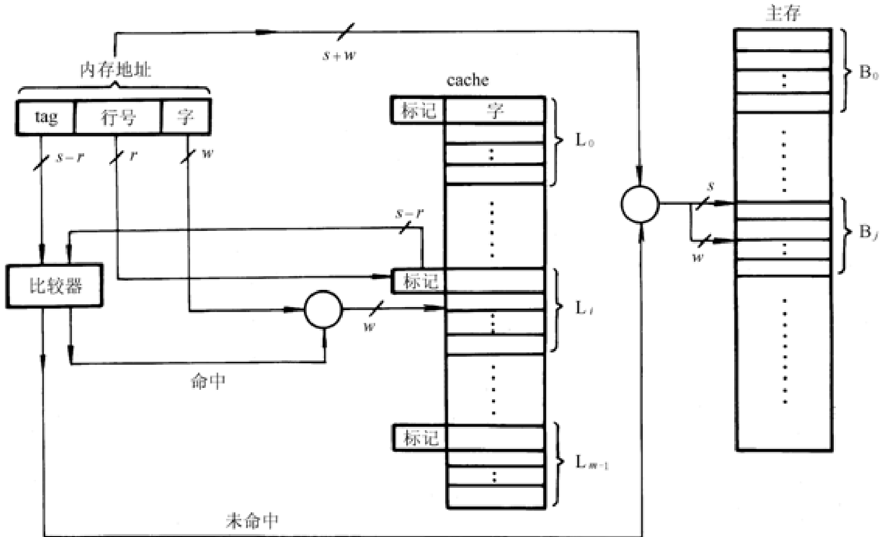
(b) 直接映射cache的检索过程
